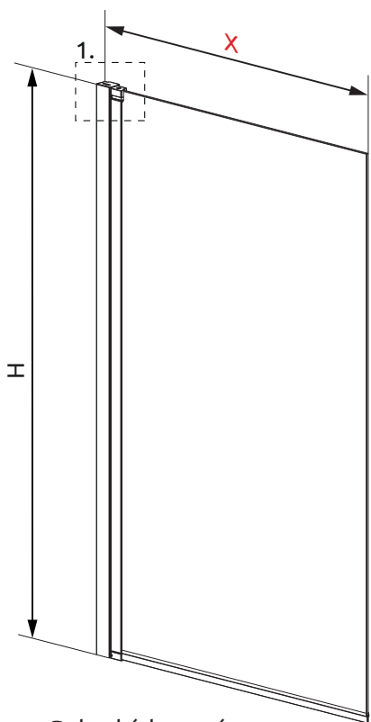
Balos kádparaván Variant L
