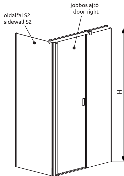
Jobbos zuhanykabin Variant R
