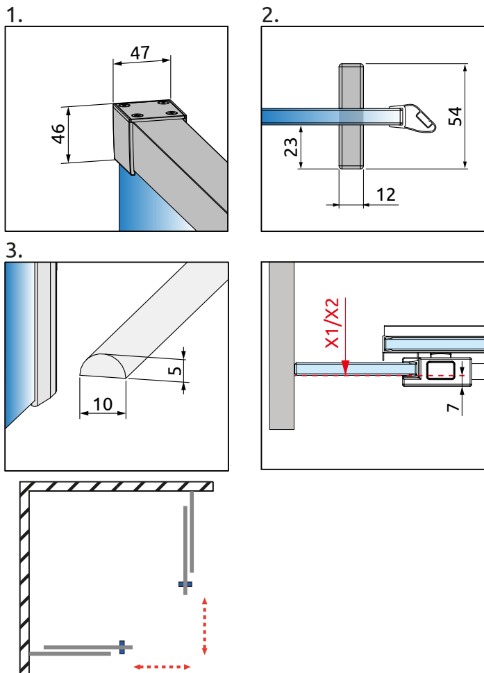
Normál méret - zuhanytálca-ra történő beépítés Standard size - assembly on a shower tray
