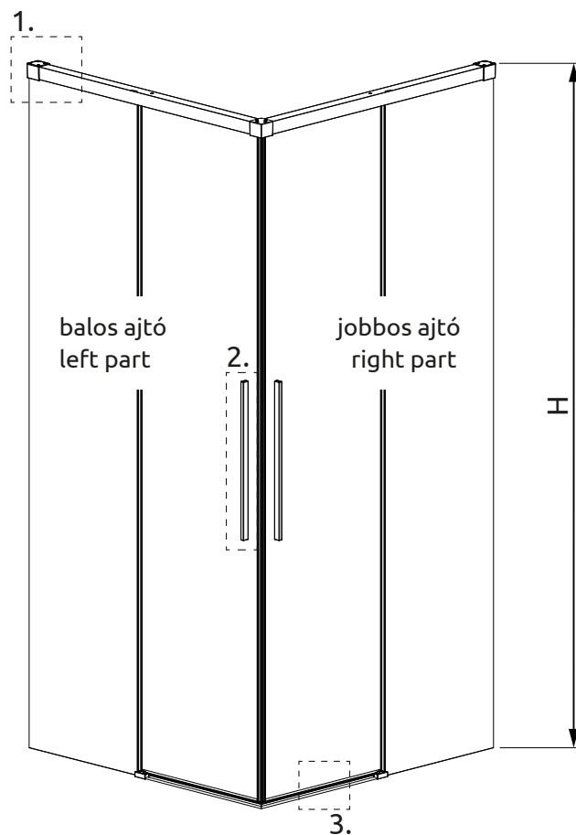
XL méret - zuhanytálca nélküli beépítés XL size - assembly without a shower tray
